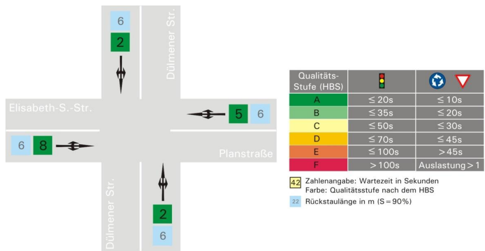
Abb. 9 Ergebnis der Leistungsfähigkeitsbetrachtungen für einen vorfahrtsregelerten Knotenpunkt
