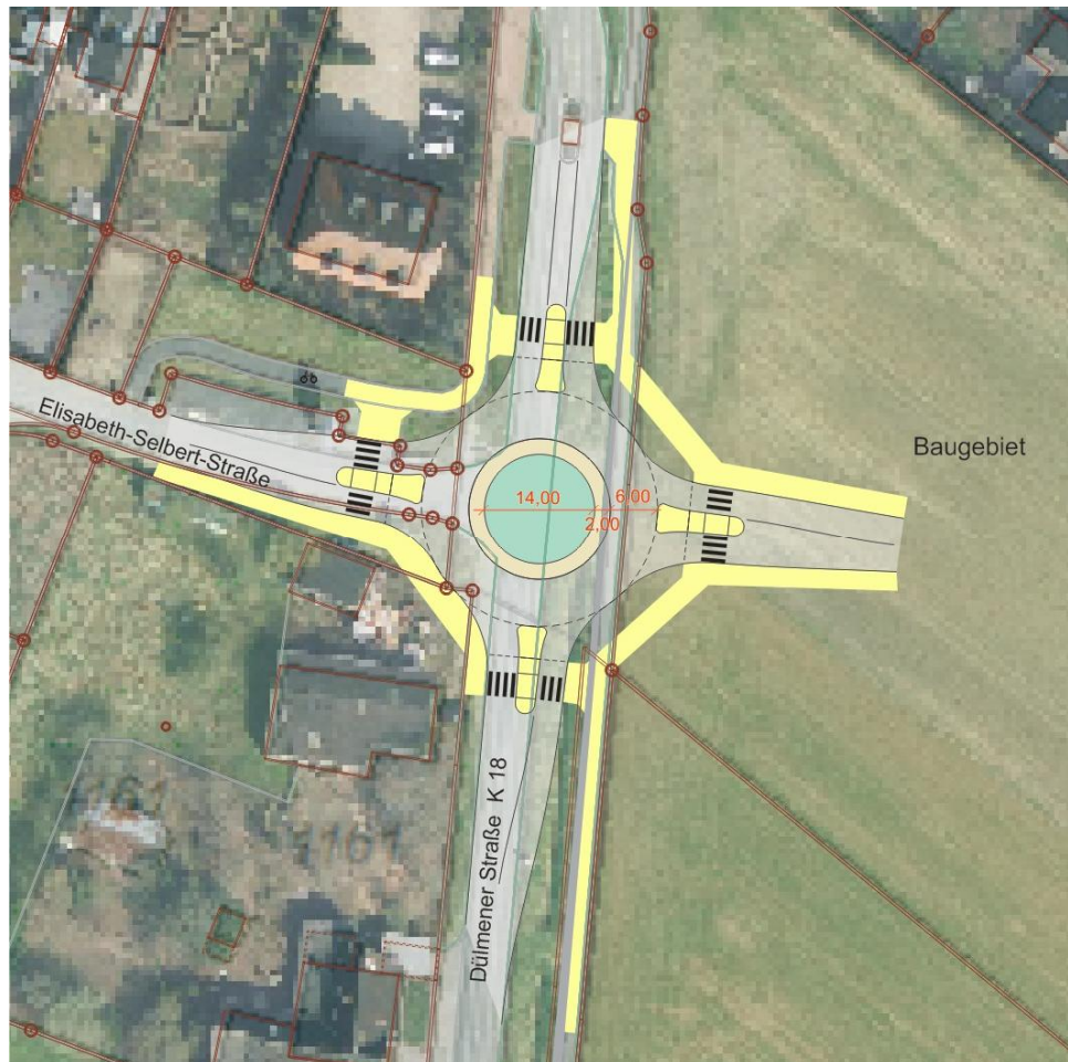
Abb. 8 Anbindung des Baugebiets an das übergeordnete Straßennetz mit einem Kreisverkehr
