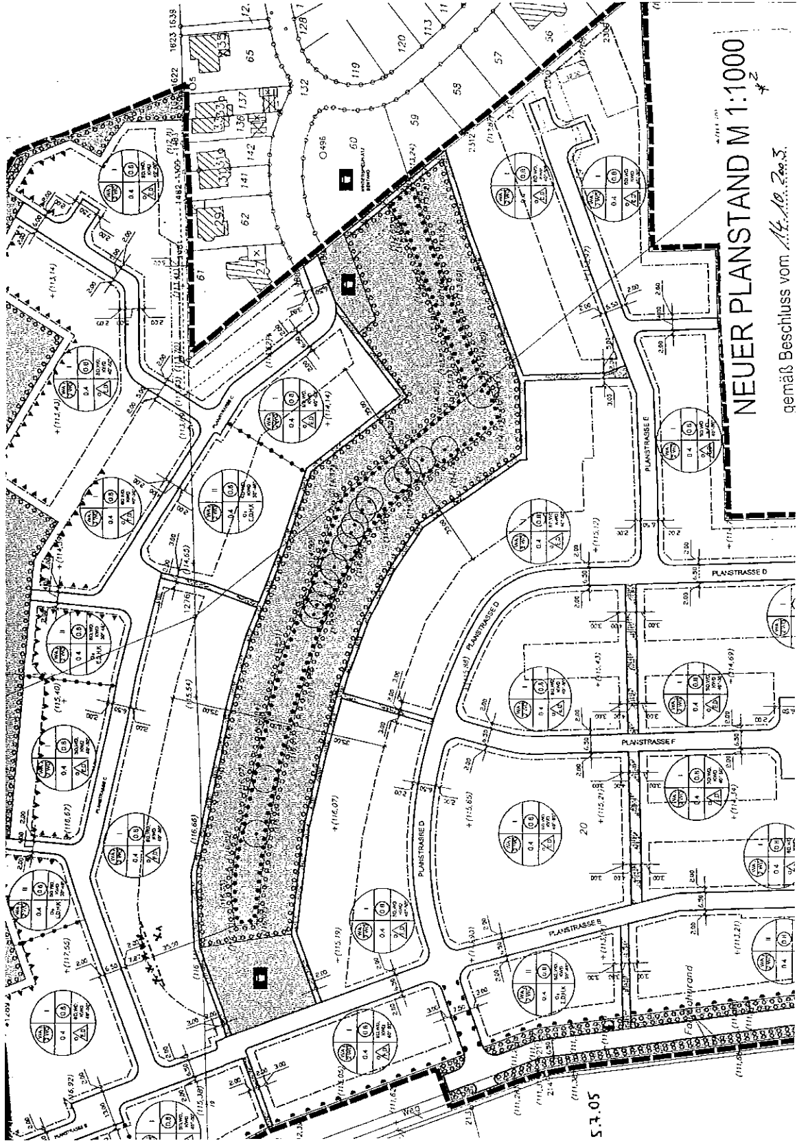
Bebauungsplan alt
